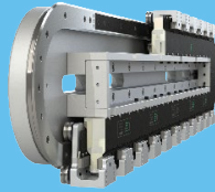
GFX 海普克公司的GFX导轨系统， 可和倍福公司的XTS 电气系统配合
