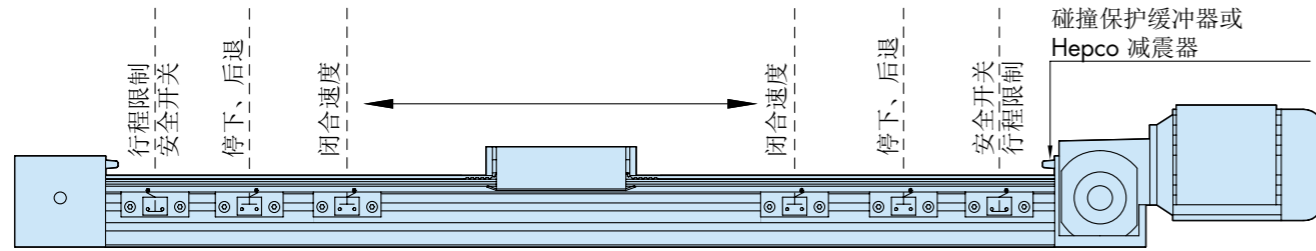
速度控制器 5
