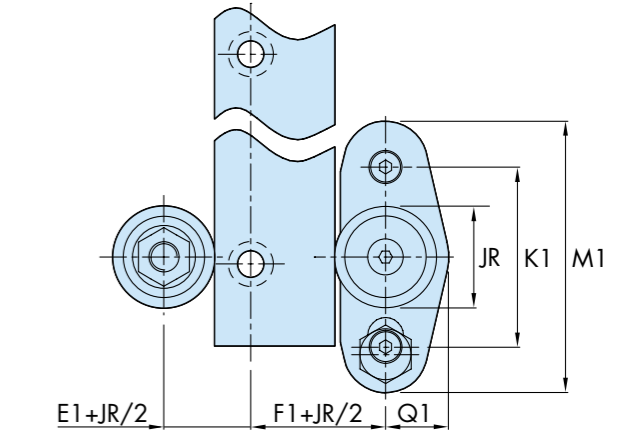
带盲孔固定轨道滚轮的平轨道
