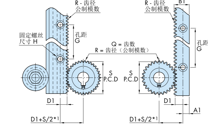
带有 V 形轴承和小齿轮的单沿垫片导轨
