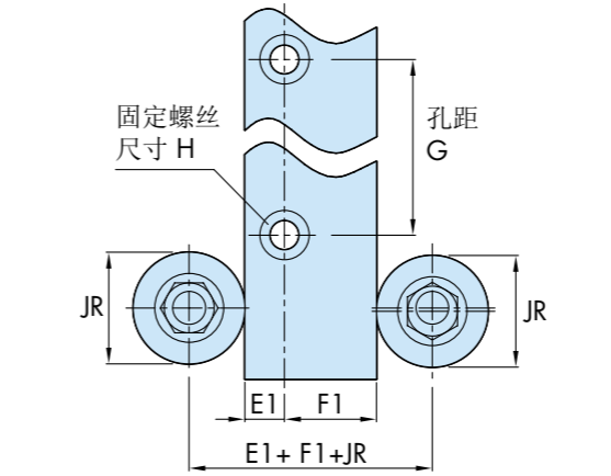
带通孔固定轨道滚轮的平轨道
